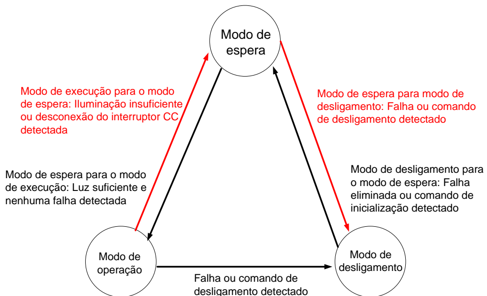
Figura 2-2 Modo operacional
