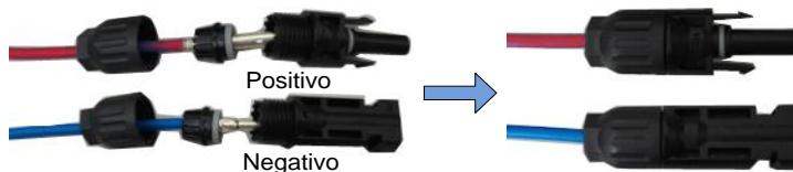
Figura 3-15 Montagem do conector
