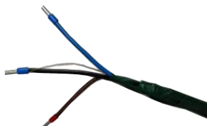
Figura 3-6 Esquema do cabo de comunicação RS485
