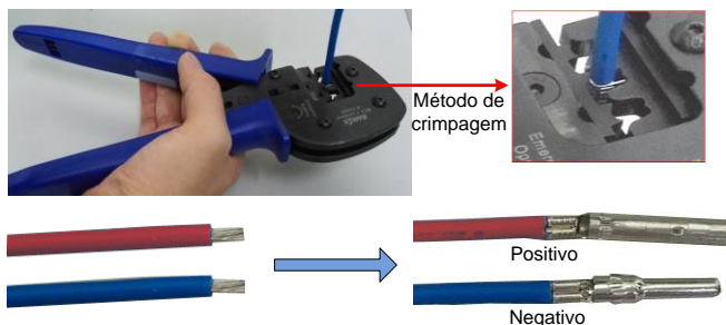
Figura 3-14 Terminal de crimpagem
