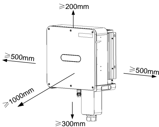
Figura 3-1 Espaço para instalação do inversor string
