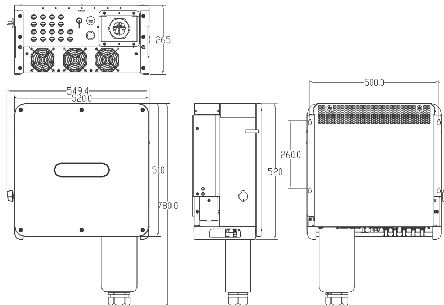
Figura 2-1 dimensões estruturais da série hopeSun (unidade: mm)
