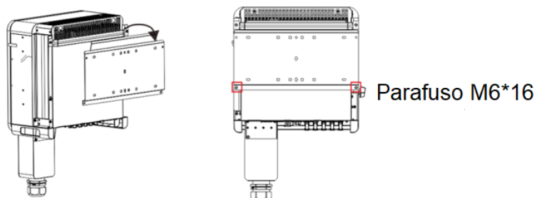
Figura 3-4 Diagrama de montagem na parede do inversor string
