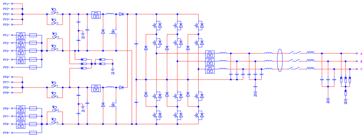
Figura 2-1 Diagrama esquemático
