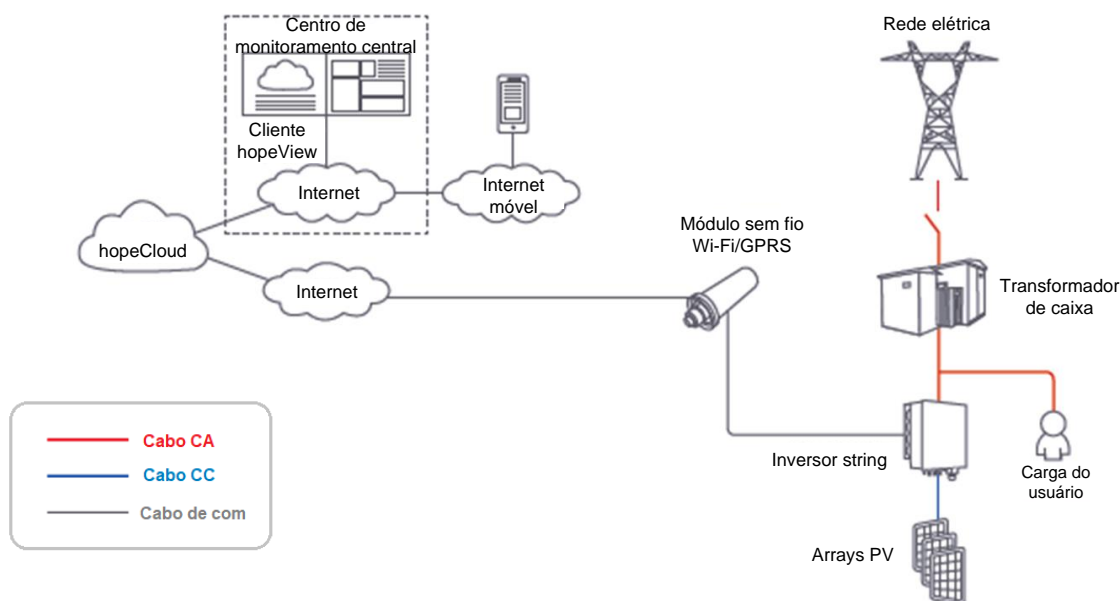
Figura 2-4 Projeto de rede de usina de energia fotovoltaica distribuída
