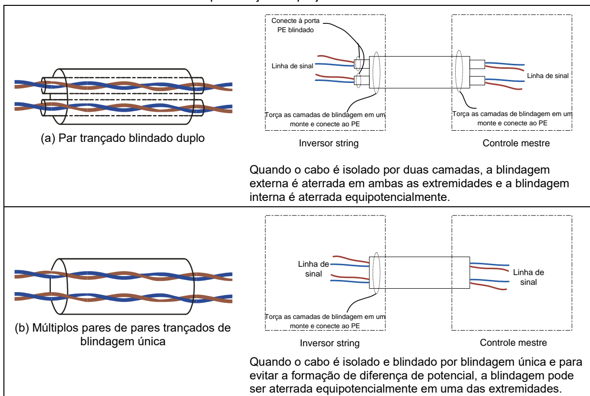
Figura 3-5 Par trançado com blindagem
