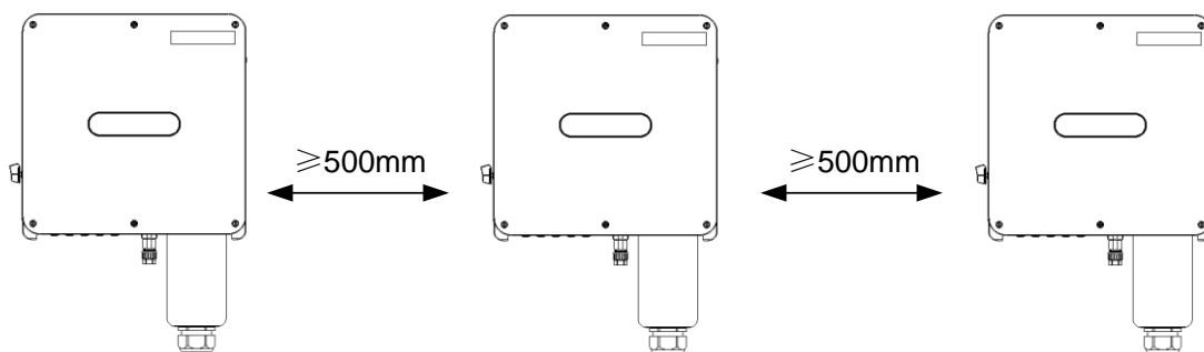
Figura 3-2 Espaço para instalação de inversores string lado a lado
