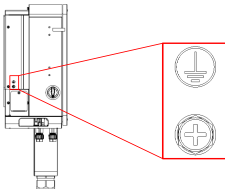
Figura 3-7 Aterramento de proteção
