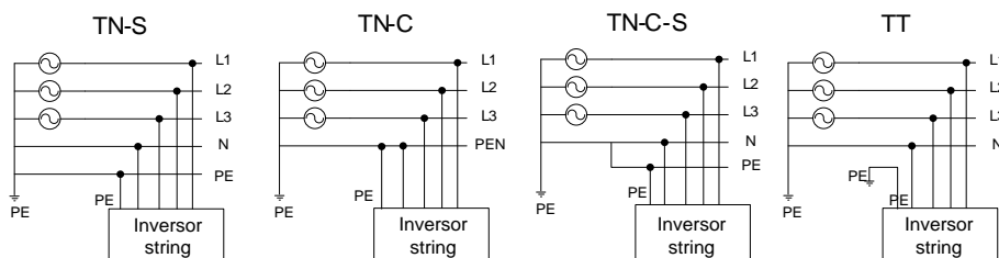
Figura 2-5 Diagrama esquemático de várias formas de rede
