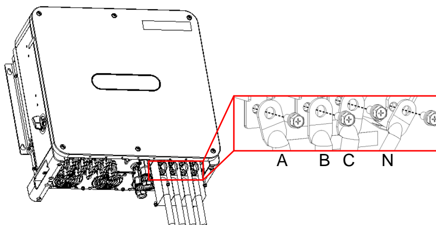
Figura 3-10 Conexão do bloco terminal CA
