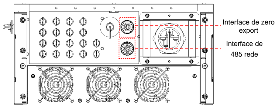
Figura 3-12 Localização das interfaces RS485 e zero export
