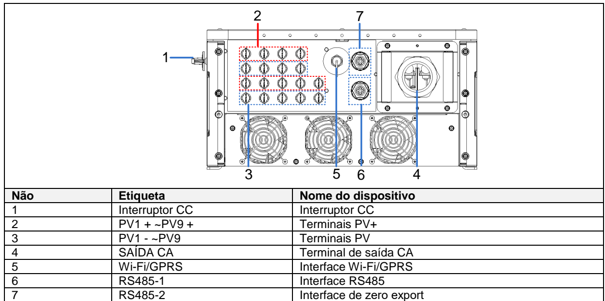
Figura 2-8 O diagrama inferior de toda a máquina (descrição da interface)
