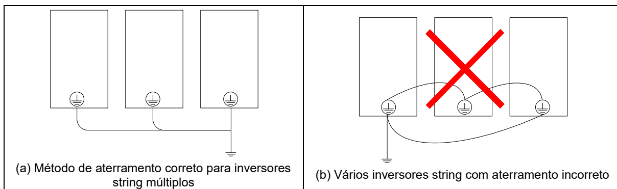
Figura 3-8 Aterramento do inversor string múltiplo
