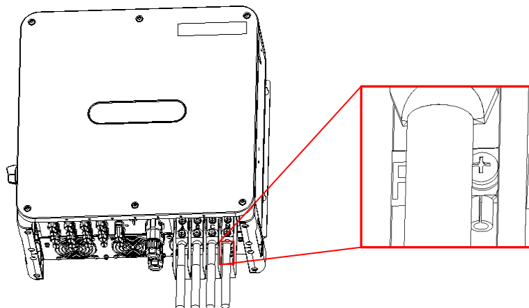
Figura 3-11 Terminal de conexão à terra do lado CA
