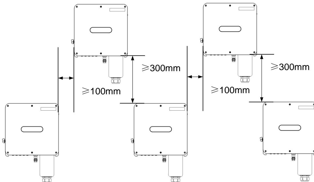
Figura 3-3 Espaço para instalação de triângulo de inversores string
