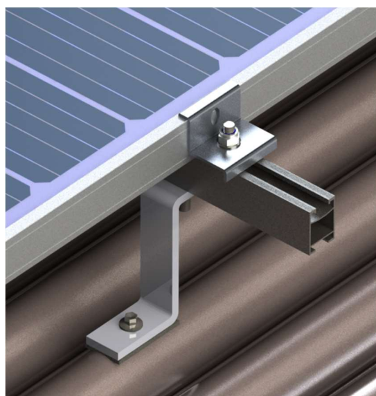
MONTAGEM DO SUPORTE E GRAMPO FINAL
