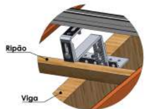
DETALHE "I" IMAGEM ILUSTRATIVA DE FIXAÇÃO
