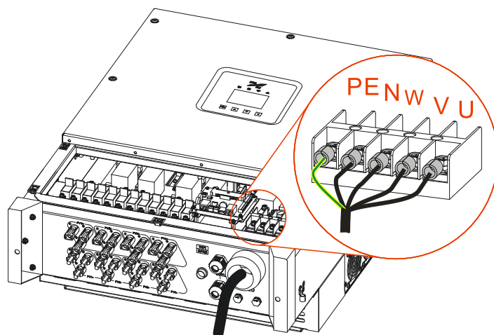
Figura 3-22 Diagrama de fiação de cabos CA
