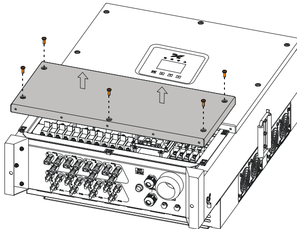
Figura 3-23 Desmonte a tampa
