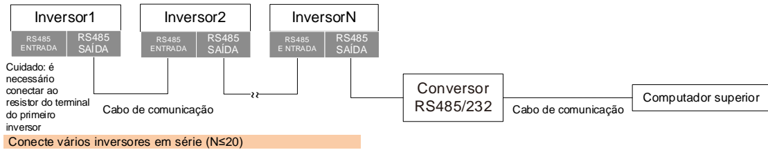
Figura 3-27 Sistema de comunicação de múltiplos inversores
