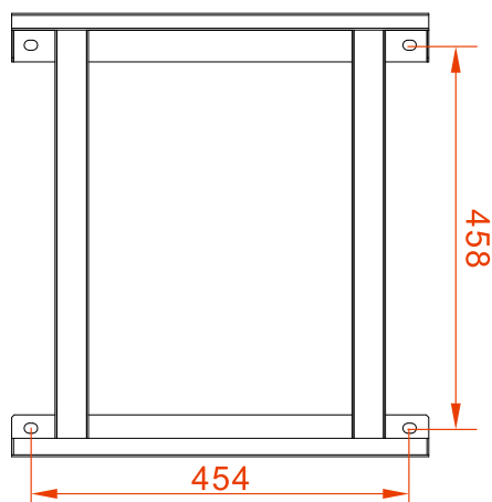
Figura 3-3 As dimensões dos furos de instalação do suporte de instalação (Unidade: mm)
