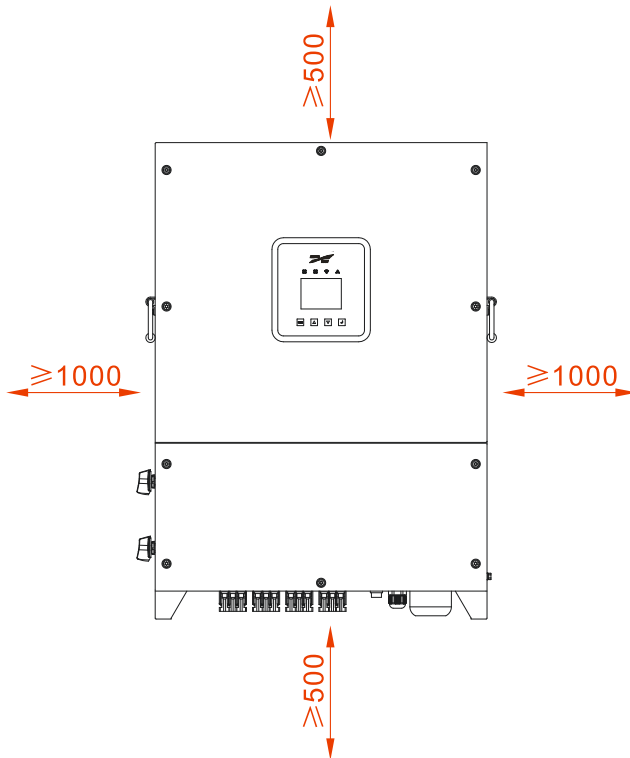
Figura 3-2 Afastamentos para instalação
