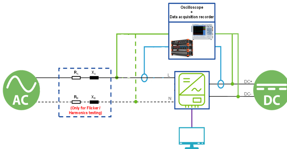
Figura 1 – Configuração do ensaio 1
