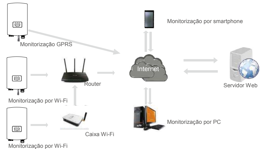
▲ Figura 4.21 Função de comunicação Wi-Fi
