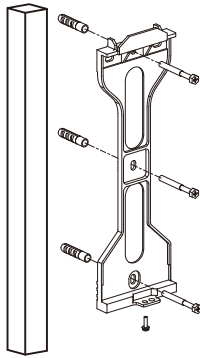
▲ Figura 4.5 Montagem do pilar do inversor
